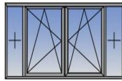
Doppio anta con fisso laterale
